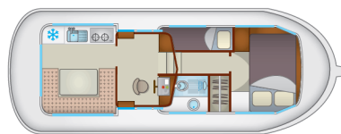
Pénichettes® 935 / 935W
